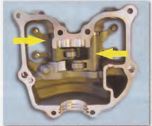
Culatín (tapa de culata) con balancines
